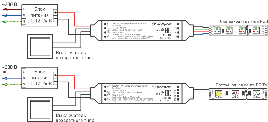
Рисунок 1. Схема подключения контроллеров SMART-K46-RGB-PUSH-SUF и SMART-K48-RGBW-PUSH-SUF
