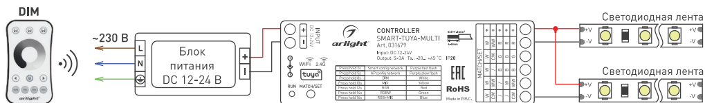
Рисунок 1. Схема подключения контроллера SMART-TUYA-MULTI
