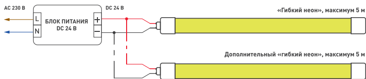
Схема 1. Подключение «гибкого неона»
